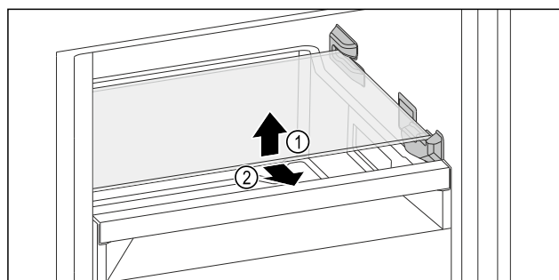
Fig. 120 Przykładowa prezentacja płyty szklanej
