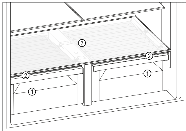
Fig. 103 Przykładowa prezentacja pokrywa komory EasyFresh (1) Komora EasyFresh (3) Półka (2) Pokrywa komory Easy-Fresh
